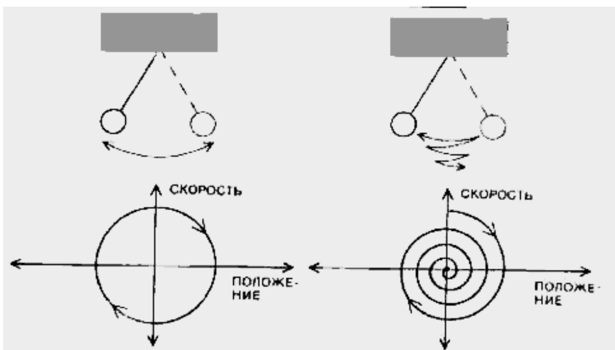
Рис.5. Линейный и нелинейный маятники и их аттракторы.
