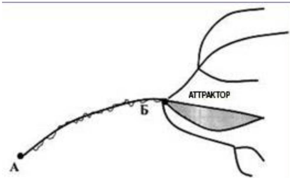
Рис.3. Схема выхода на аттрактор.
