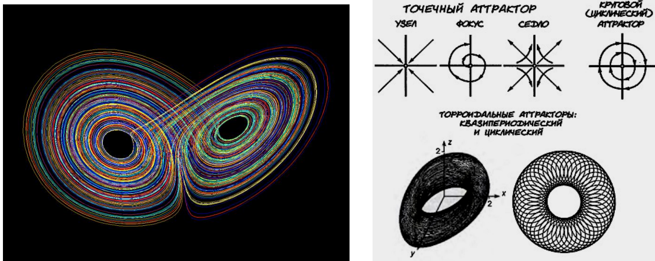
Рис. 8 Вид странного аттрактора Лоренца (слева) и виды простых аттракторов (справа).
